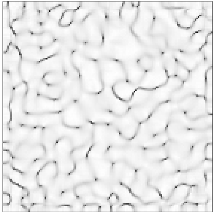
(b) Gradient
