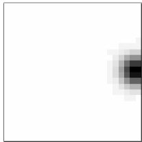
(d) Iteration 40,000
