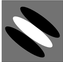
(d) 3-lobe V1 simple cell
