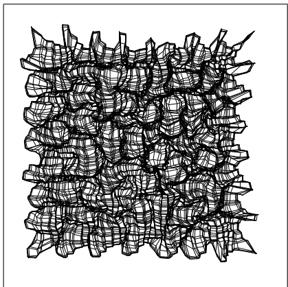
(b) Retinotopy
